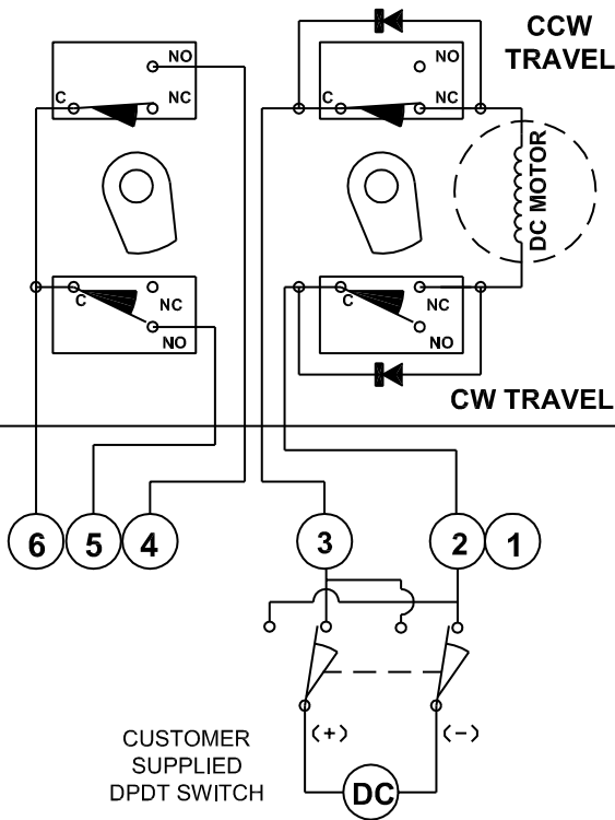
WIRING SCHEMATIC
